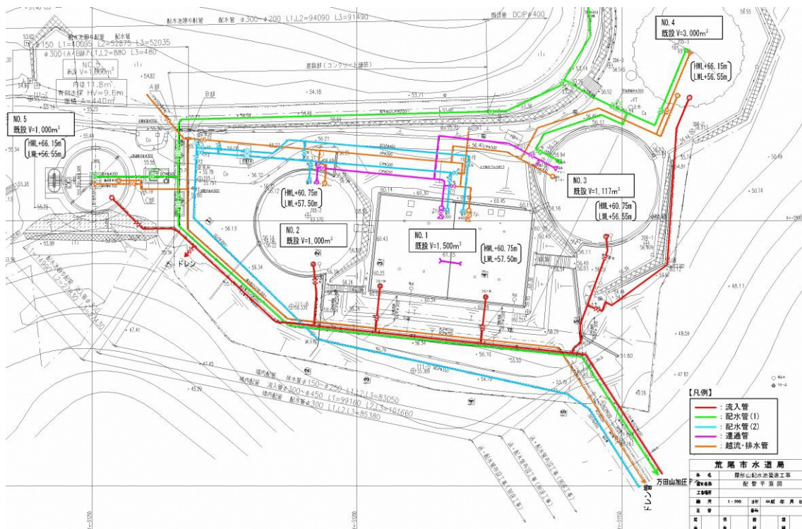
図 2-1 屋形山配水池平面図
