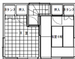
2階平面図
