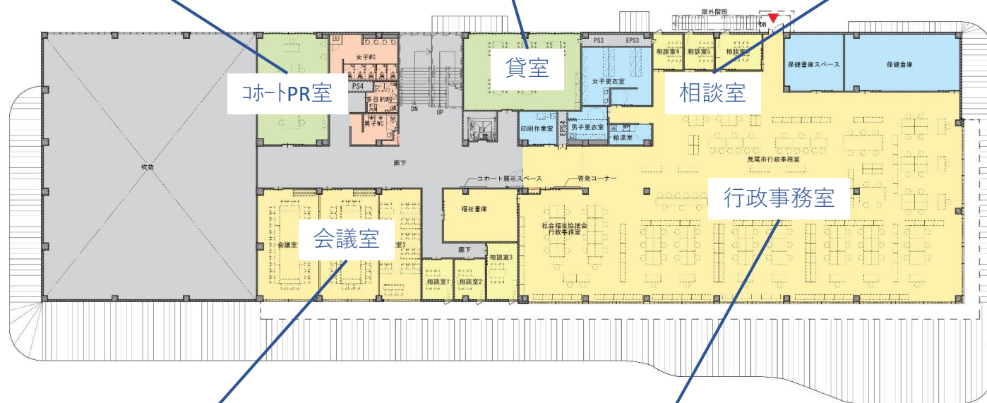
2 階平面図
