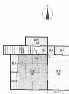
2階 縮尺 1/100
