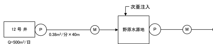
図 6.4 野原水源系フロー
