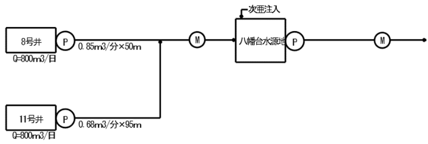
図6.2 八幡台水源池フロー
