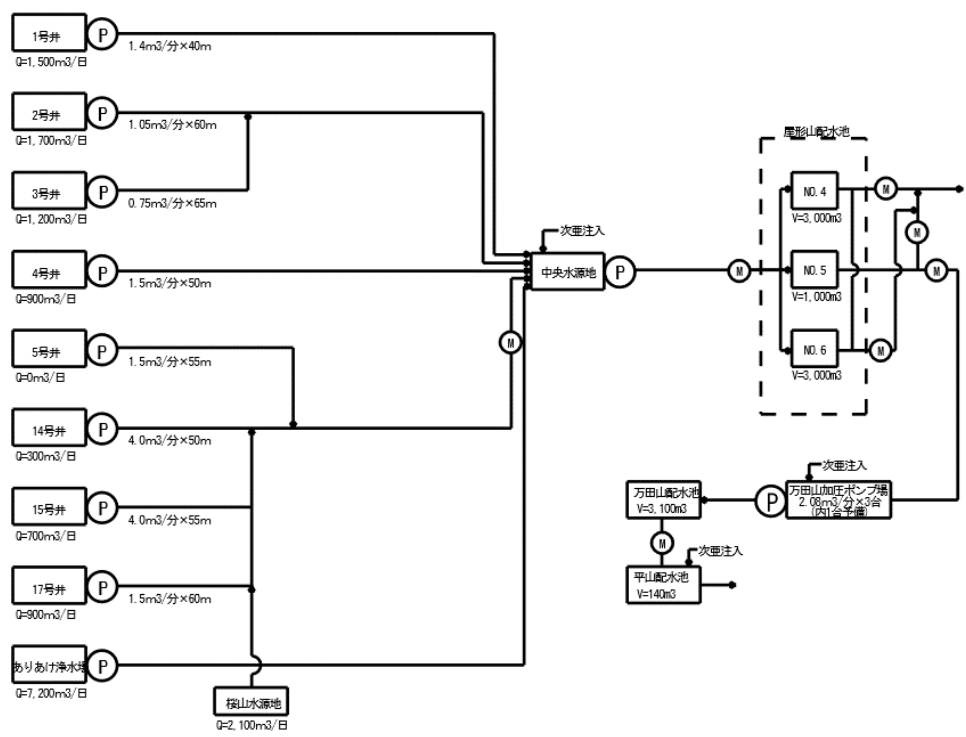
図6.1 中央水源系フロー
